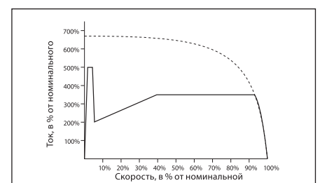
Кратковременный ток и нарастание тока при использовании импульсного пуска
